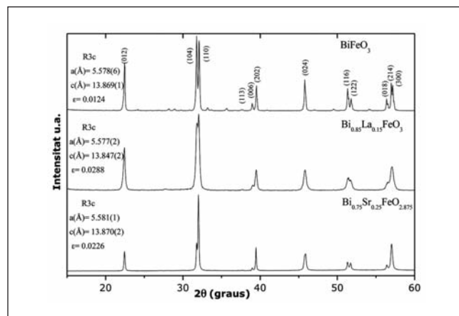
Figura 5. Diagrames de difracció de raigs X corresponents a les mostres \text{BiFeO}_3 , \text{Bi}_{0,85}\text{La}_{0,15}\text{FeO}_3 , \text{Bi}_{0,75}\text{Sr}_{0,25}\text{FeO}_{2,875} .
