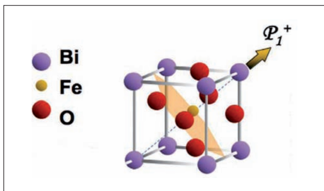
Figura 3. Cel·la unitària de tipus romboèdric de la perovskita de BiFeO 3 .
